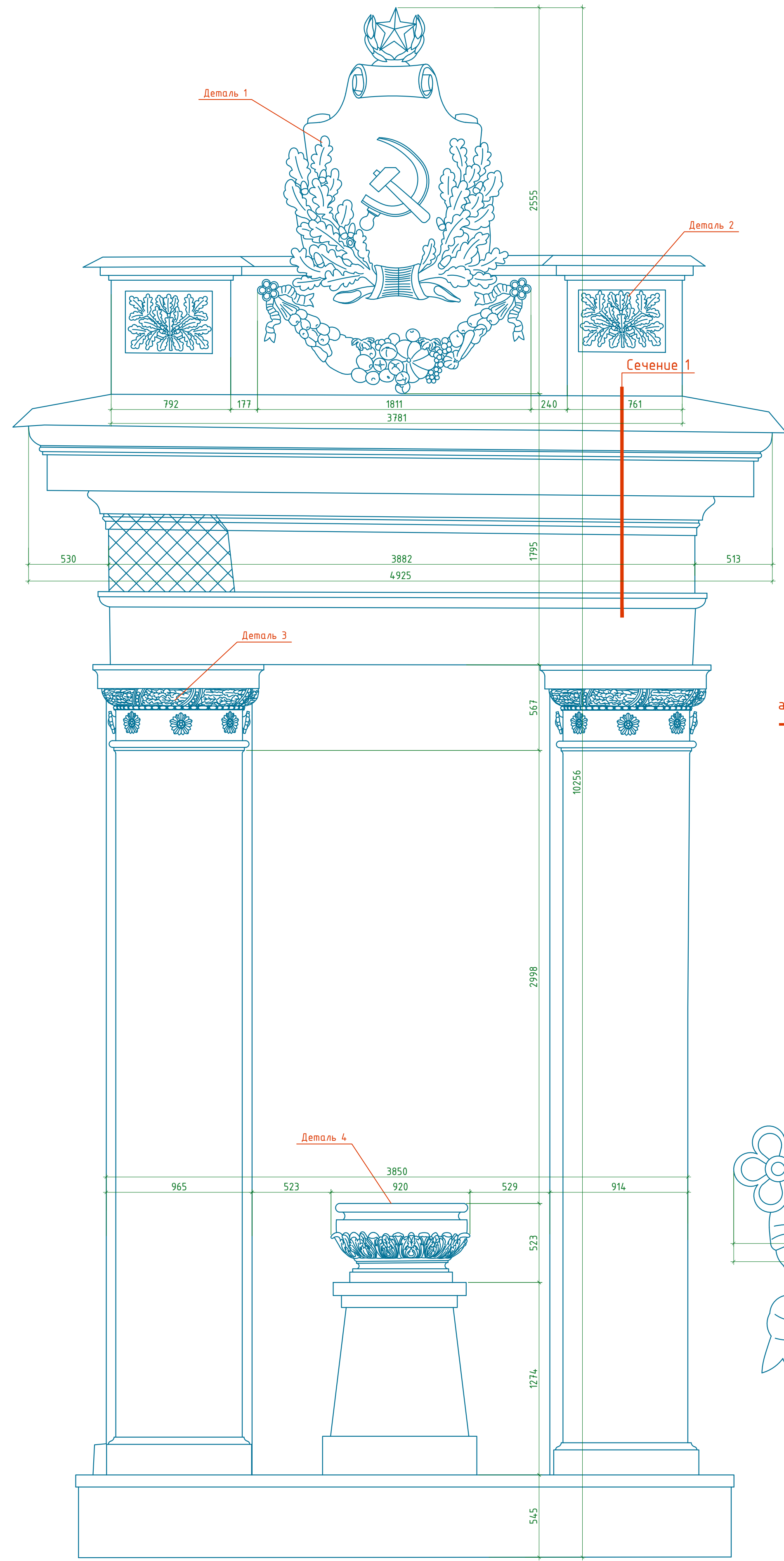
Фрагмент 1. Общий вид. М 1:20.
