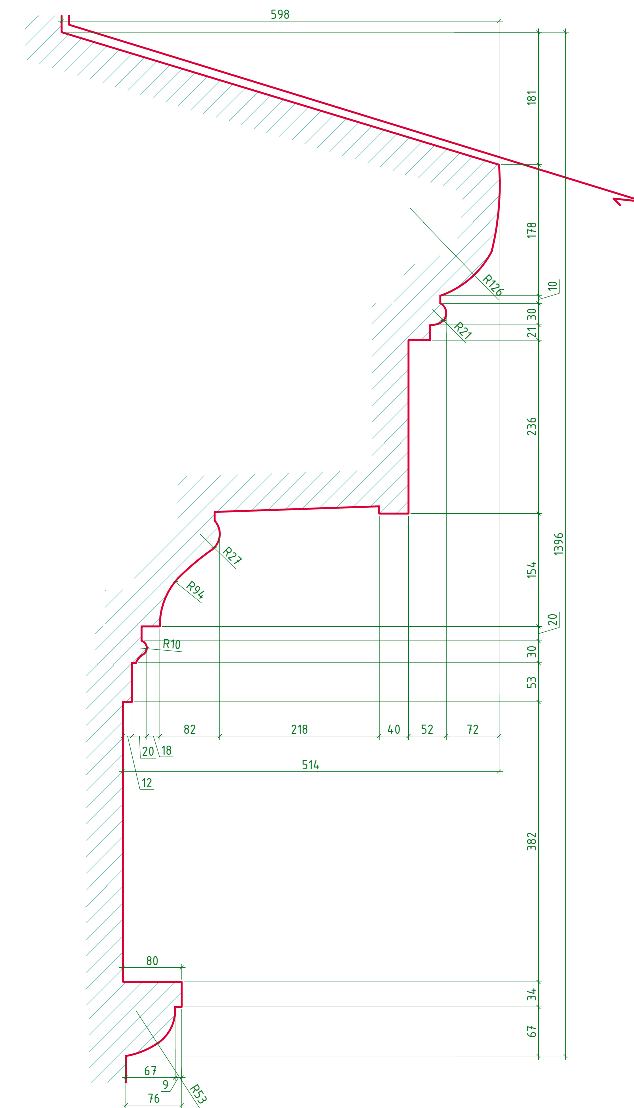
Сечение 1. М 1:5.
