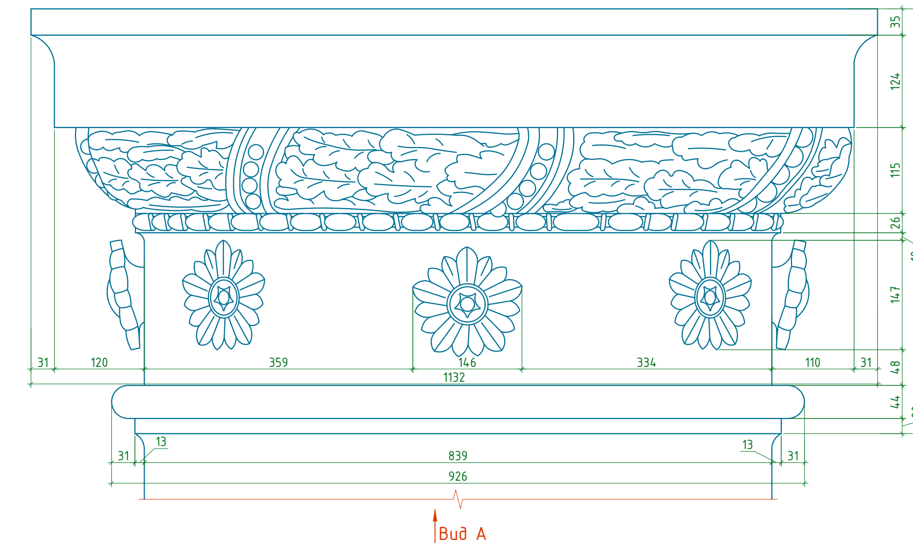
Вид А. М 1:5.
