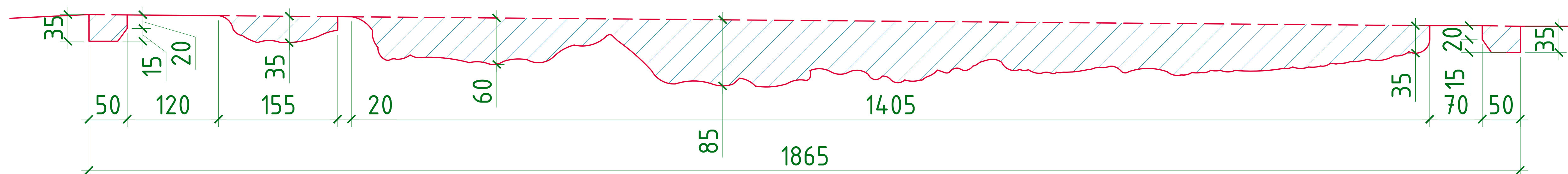
Сечение а-а. М 1:10
