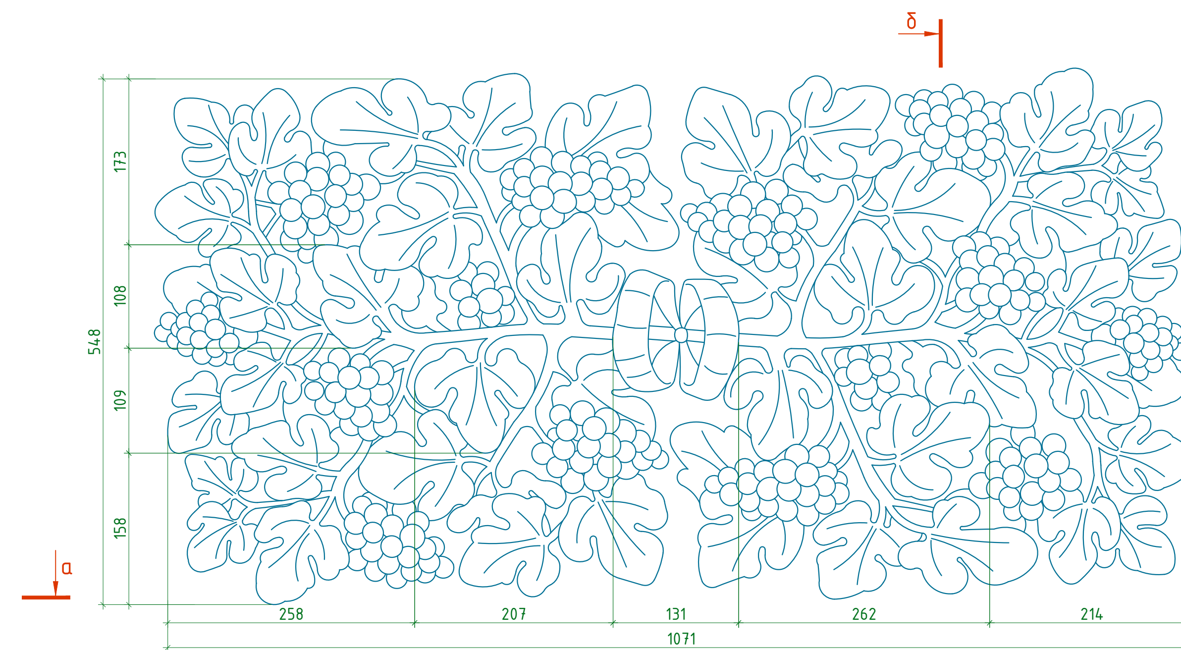
Деталь 2. Общий вид. М 1:5.
