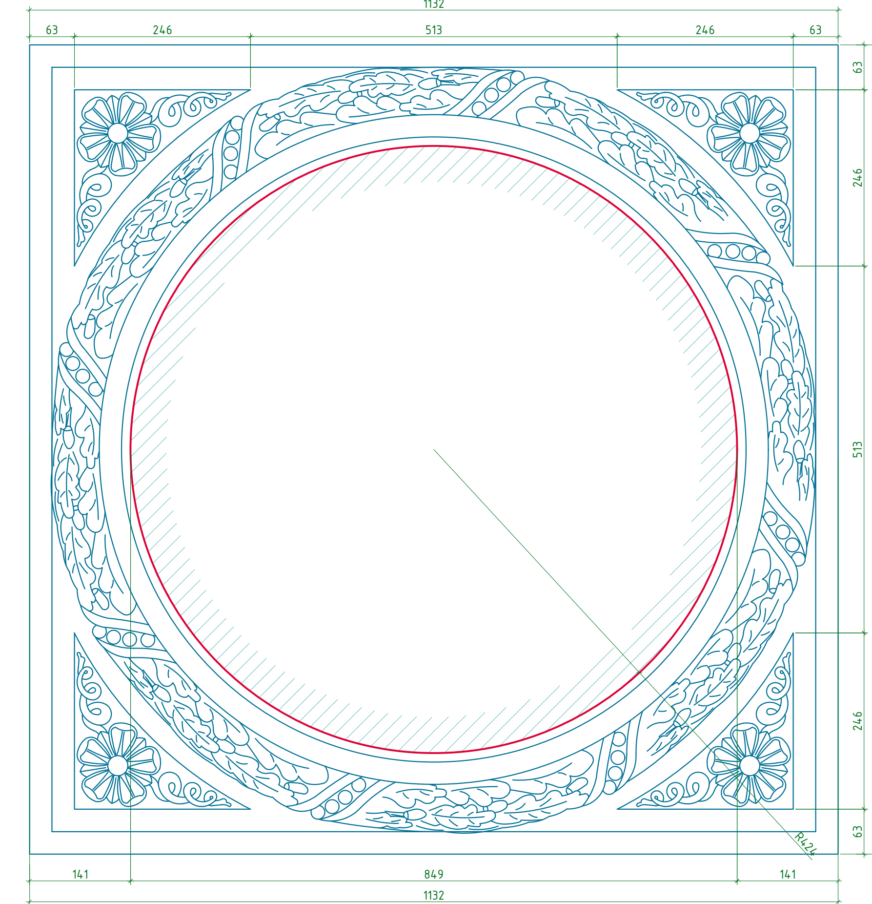
Вид А. М 1:5.
