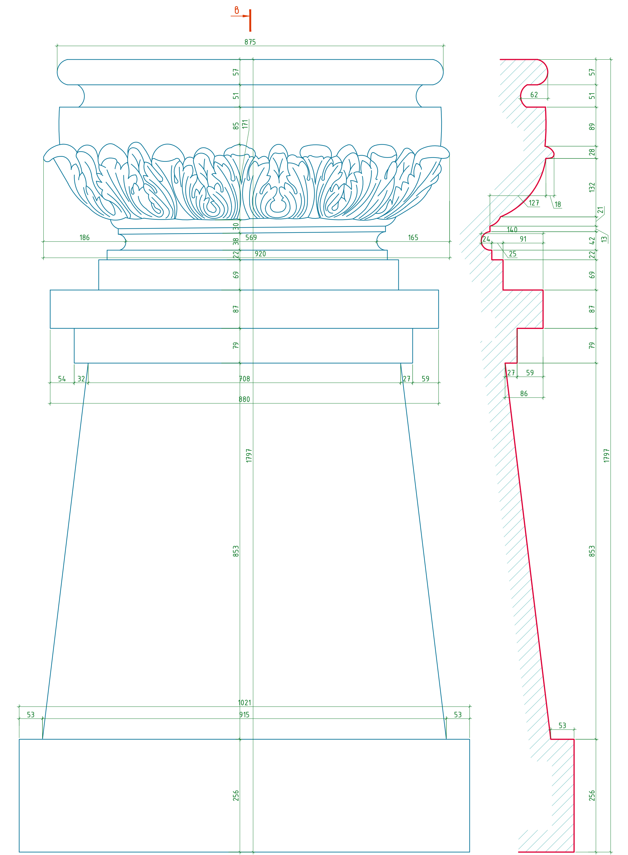
Деталь 4. Общий вид. М 1:5.
