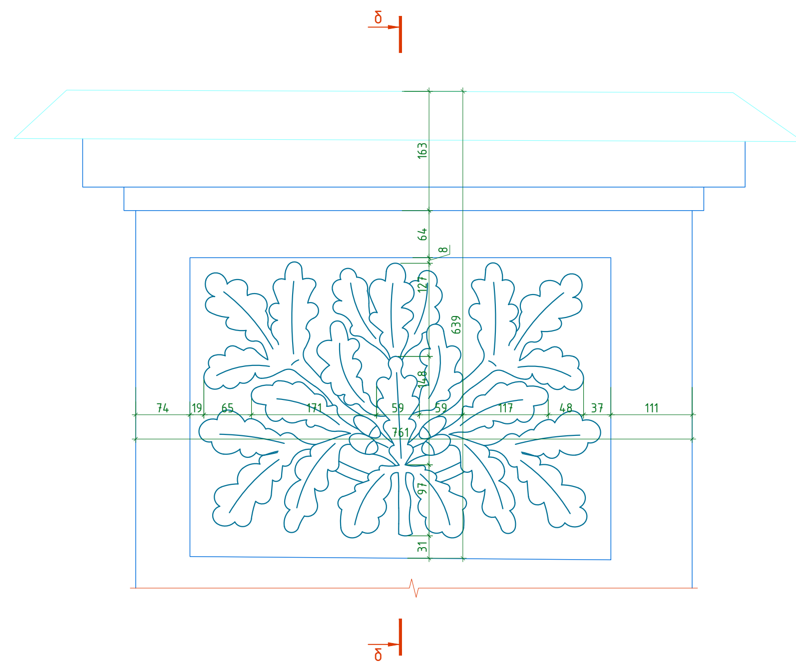
Деталь 2. Общий вид. М 1:5.
