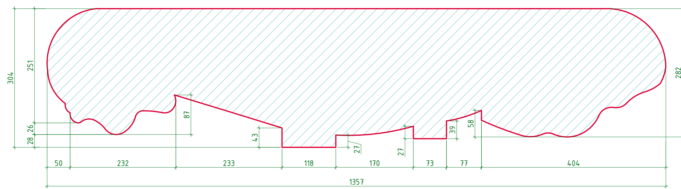
а-а
