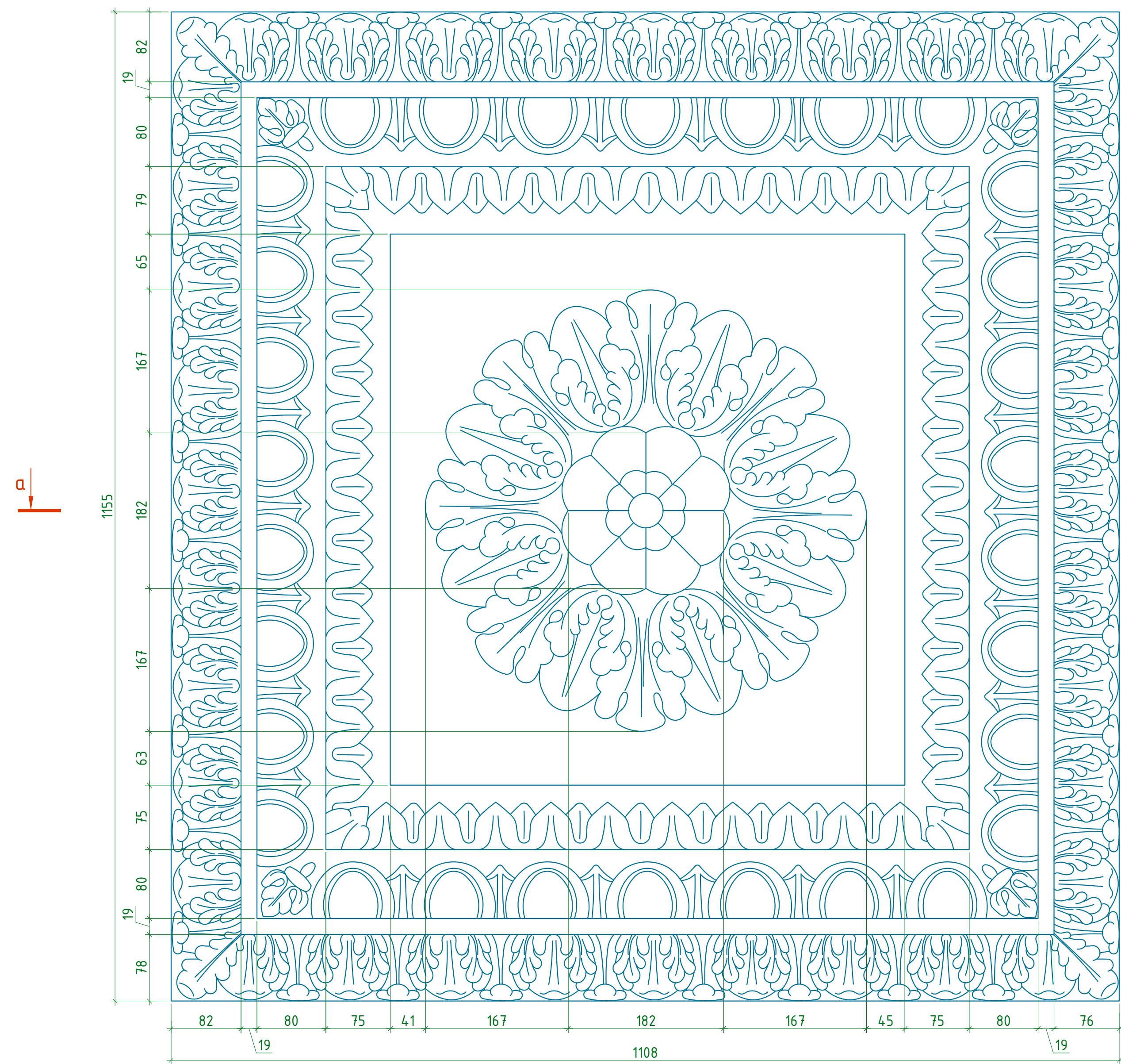
Деталь 1. Общий вид. М 1:5.
