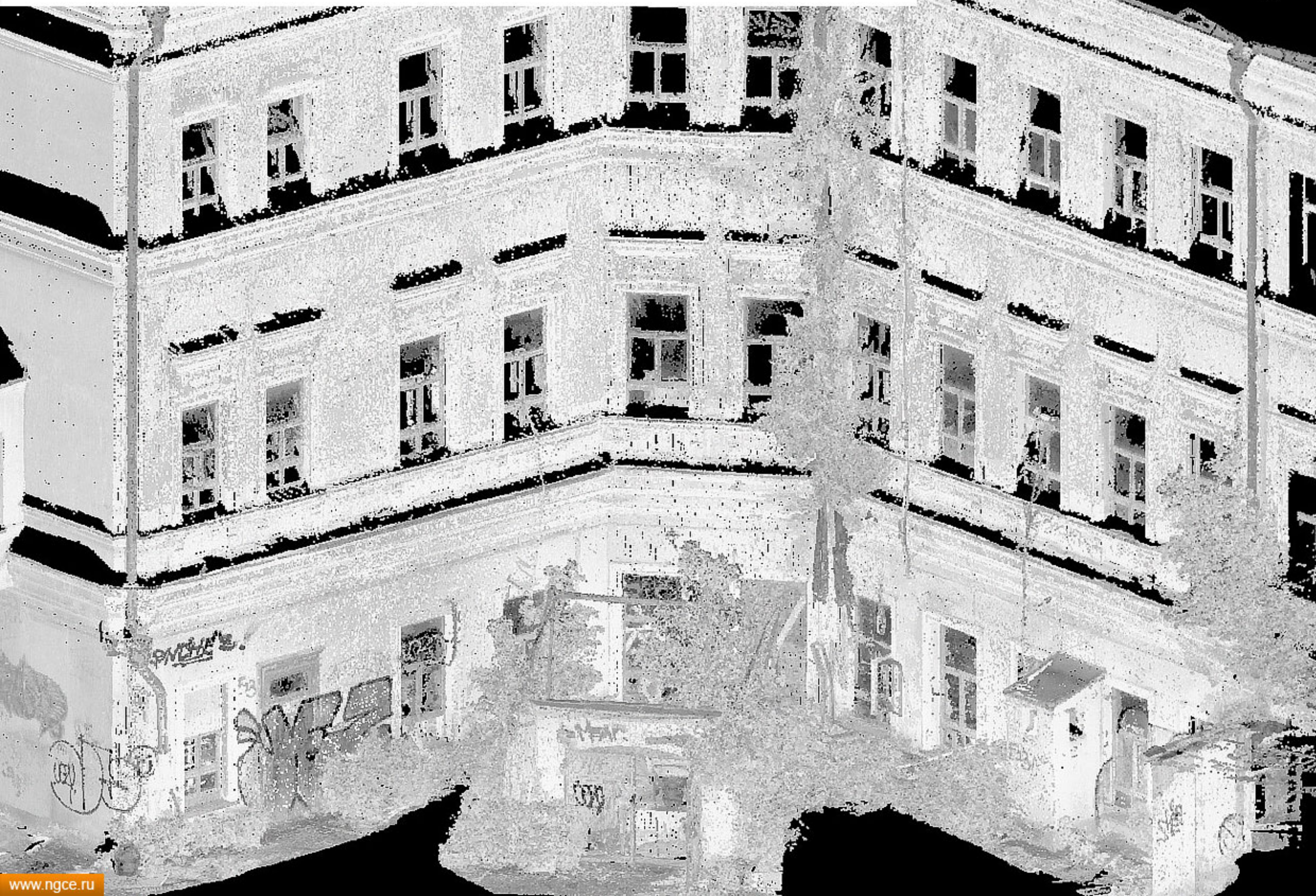
Фрагмент облака точек заднего фасада «Дома с атлантами», выходящего во внутренний двор
