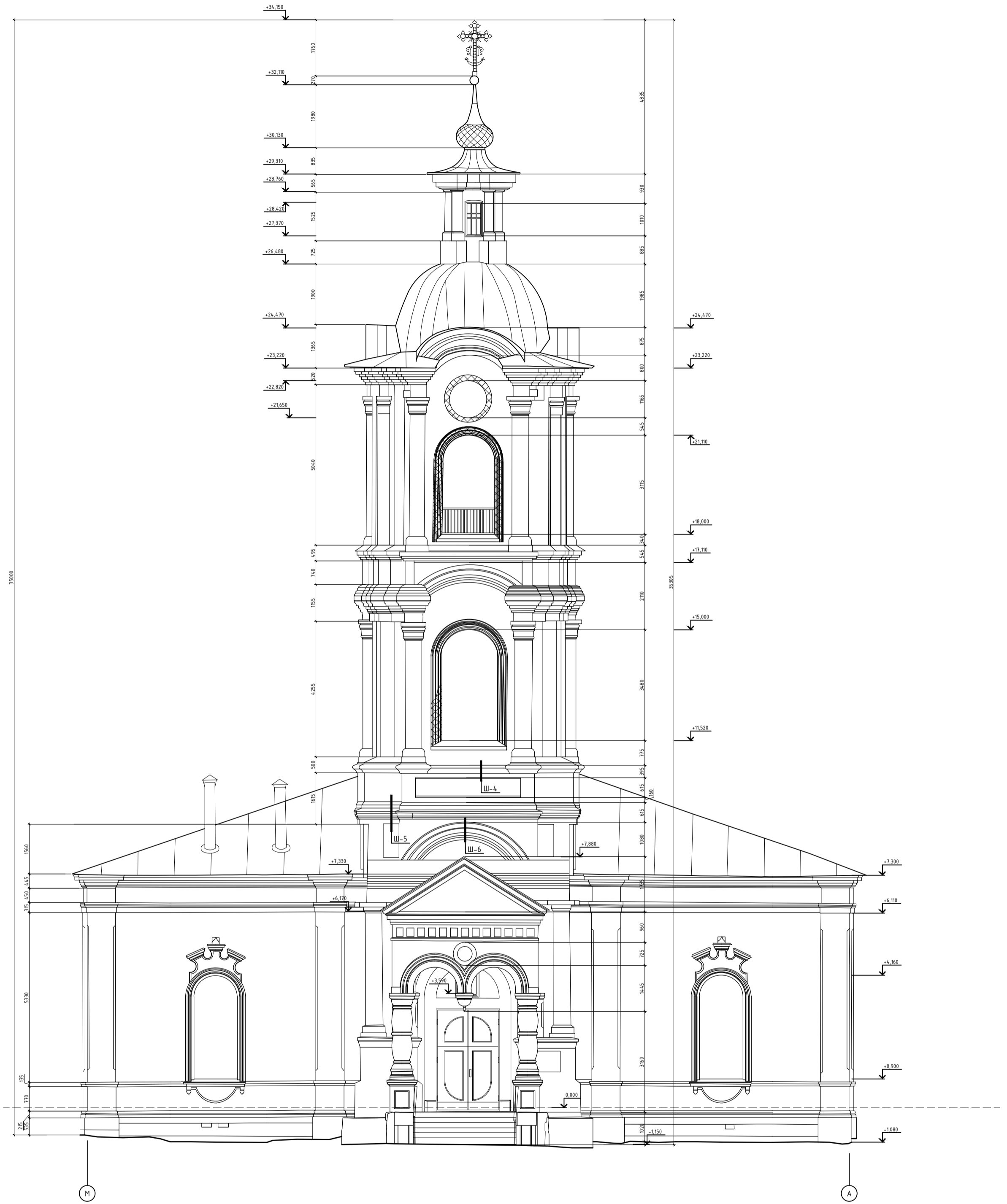
Фасад в осях М-А (Западный) М 1:50
